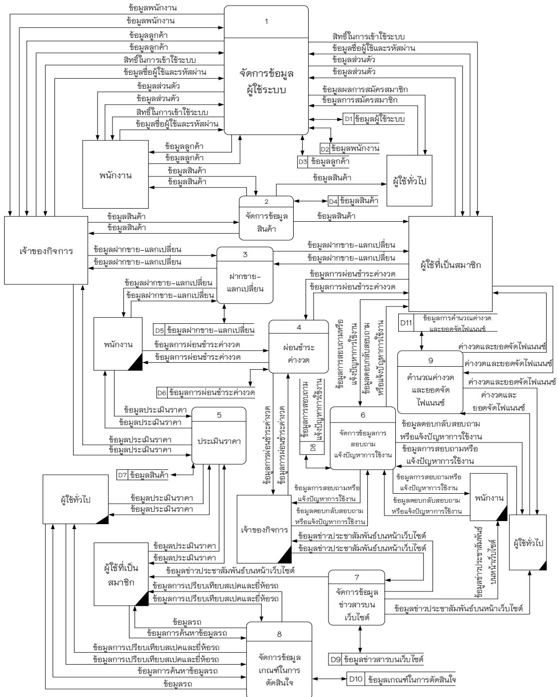
ภาพที่ 3.7 แผนภาพกระแสข้อมูลระดับที่ 0 ระบบบริหารจัดการข้อมูลและสนับสนุนการตัดสินใจการเลือกซื้อรถยนต์มือสองบนเว็บไซต์ บริษัท รุ่งโรจน์59 จำกัด
